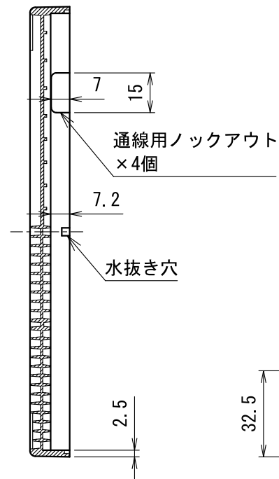
A-A断面図
